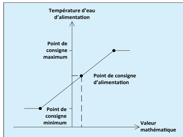
Figure 34 - Compensation par valeur mathématique
