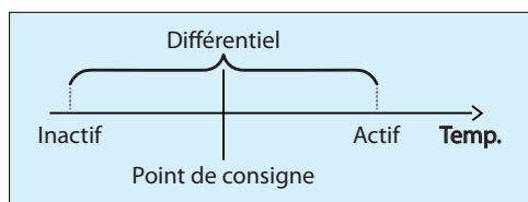
Figure 26 - Fonctionnement des étapes sur différentiel de consigne
