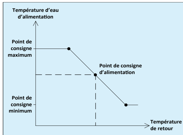
Figure 32 - Compensation par température d'eau de retour
