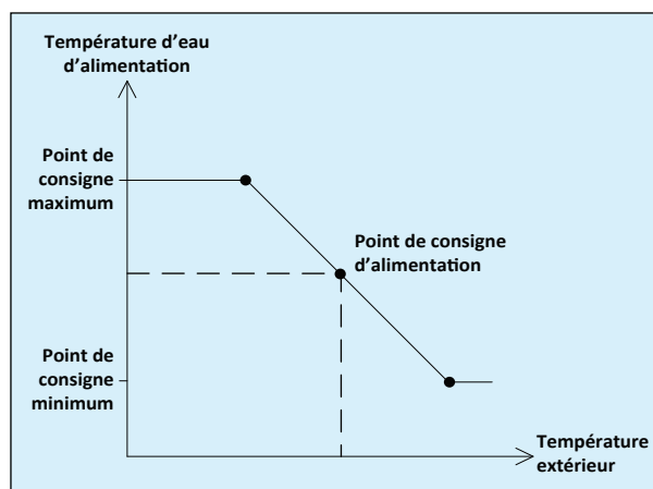
Figure 33 - Compensation par température extérieure
