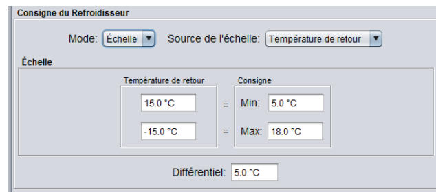
Figure 31 - Échelle de compensation de la consigne
