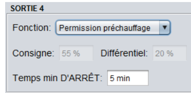
Figure 37 - Fenêtre de configuration de la sortie digitale 4
