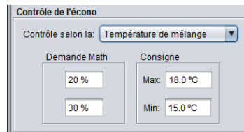
Figure 64 - Fenêtre de configuration de la température de mélange de l'économiseur
