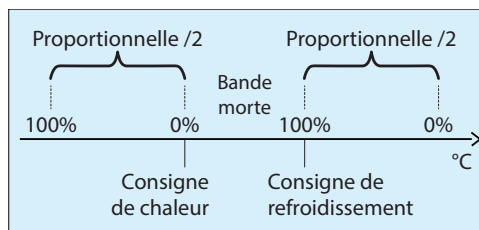
Figure 54 - Fenêtre de bande proportionnelle de boucle PI
