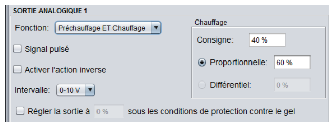
Figure 42 - Fenêtre de configuration de la sortie analogique 1
