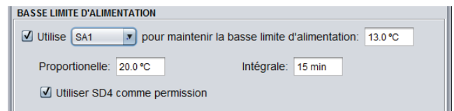
Figure 50 - Basse limite d'alimentation - contrôle de sortie analogique
