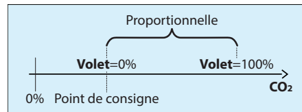
Figure 70 - Fenêtre de bande proportionnelle de CO 2
