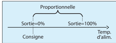
Figure 34 - Composante proportionnelle de la boucle PI du refroidissement analogique
