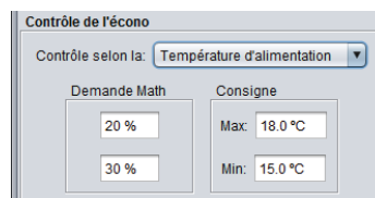
Figure 63 - Fenêtre de configuration de la température d'alimentation de l'économiseur
