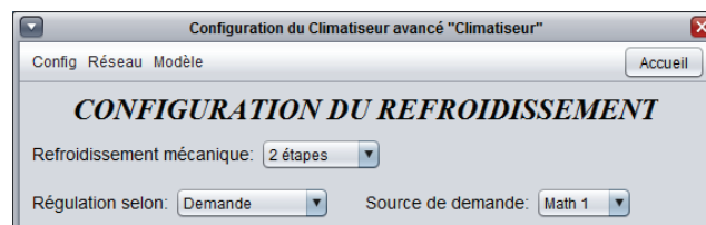
Figure 23 - Configuration du refroidissement
