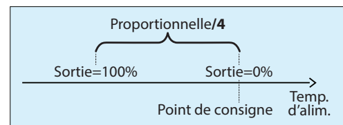
Figure 51 - Basse limite d'alimentation - bande proportionnelle analogique
