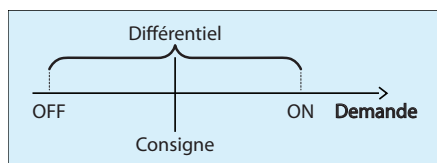
Figure 43 - Différentielle de contrôle du chauffage selon la demande
