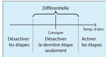
Figure 32 - Fenêtre de contrôle du refroidissement par étapes selon la température d'alimentation
