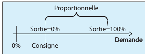
Figure 77 - Fenêtre de déshumidification analogique selon la demande
