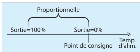
Figure 46 - Fenêtre de bande proportionnelle du préchauffage
