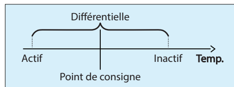
Figure 60 - Fenêtre de différentielle de consigne été/hiver de l'économiseur
