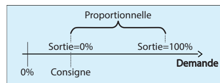
Figure 44 - Proportionnelle de contrôle du chauffage selon la demande
