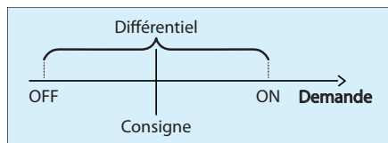
Figure 40 - Différentielle de contrôle du chauffage selon la demande
