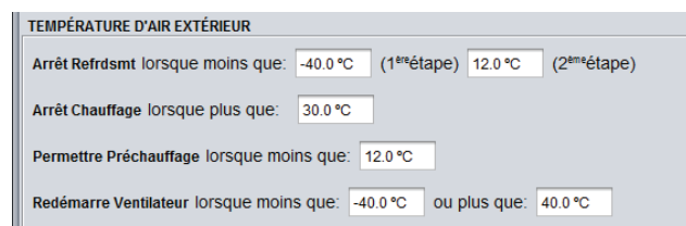
Figure 83 - Fenêtre de limites de température d'air extérieur
