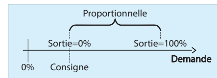
Figure 41 - Proportionnelle de contrôle du chauffage selon la demande
