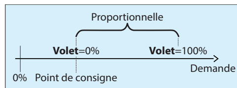
Figure 62 - Fenêtre de bande proportionnelle du volet de l'économiseur
