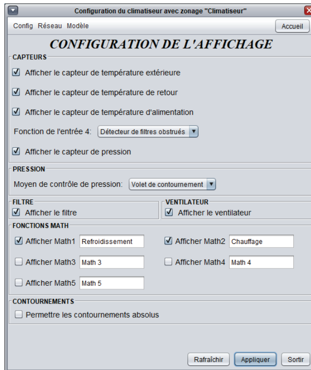
Figure 20 - Fenêtre de configuration de l'affichage
