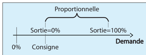
Figure 79 - Fenêtre de déshumidification de l'économiseur selon la demande
