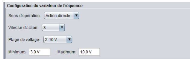
Figure 57 - Fenêtre de configuration du variateur de fréquence
