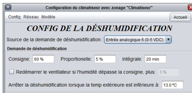
Figure 73 - Fenêtre de Configuration de déshumidification (à l'aide de l'entrée analogique 6, transmetteur d'humidité 0-5 VDC)
