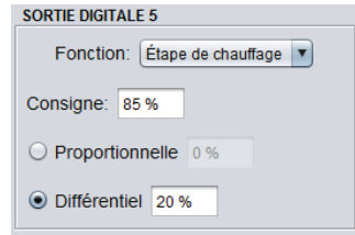
Figure 39 - Fenêtre de configuration de la sortie digitale 5
