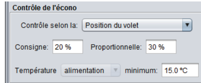
Figure 61 - Fenêtre de configuration de la position du volet de l'économiseur
