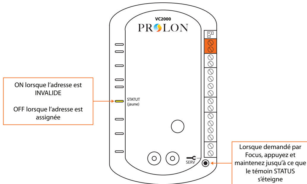
Figure 17 - Assignation d'une adresse de réseau
