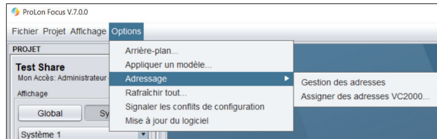
Figure 45 - Menu d'adressage
