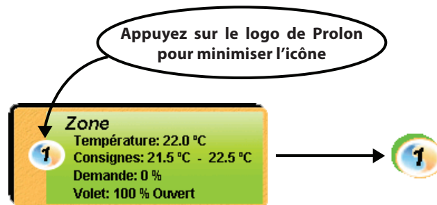
Figure 13 - Minimisation d'icône
