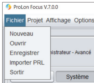
Figure 30 - Menu fichier
