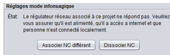
Figure 27 - Opération d'association
