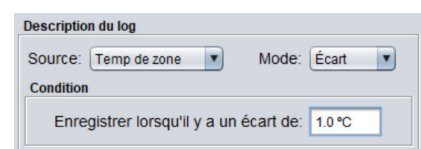
Figure 35 - Échantillonnage par écart de valeur
