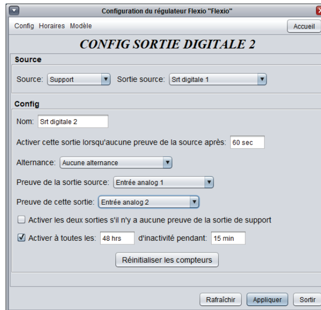
Figure 36 - Configuration de l'étape de support de la sortie
