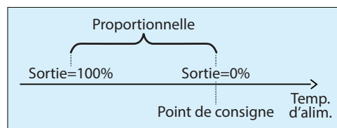
Figure 27 - Bande proportionnelle de l'air d'alimentation
