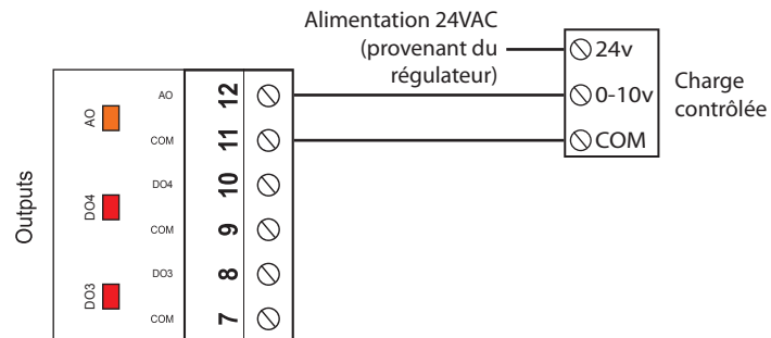
Figure 15 - Raccordement de la sortie analogique (alimenté par le régulateur)
