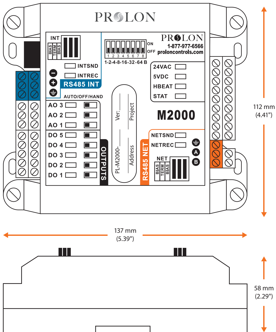
Figure 20 - Dimension du M2000
