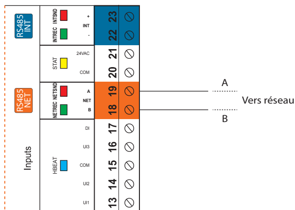
Figure 16 - Raccordement au réseau
