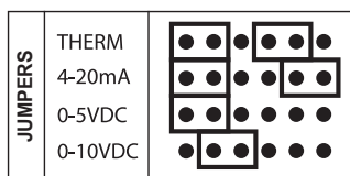
Figure 6 - Entrées analogiques
