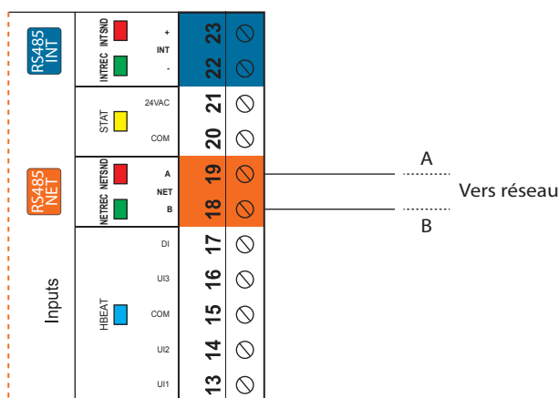
Figure 15 - Raccordement au réseau
