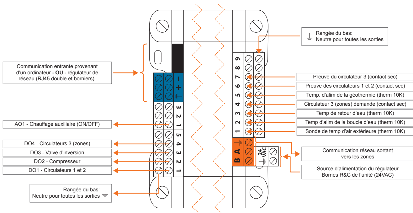
Figure 12 - Identification des entrées et sorties (boucle de chaudière ouverte)
