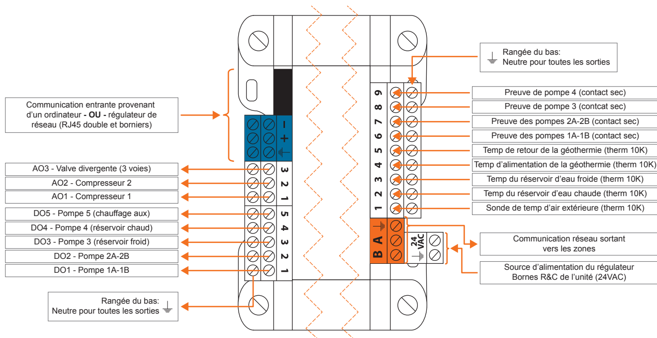
Figure 21 - Identification des entrées et sorties (récupération double)
