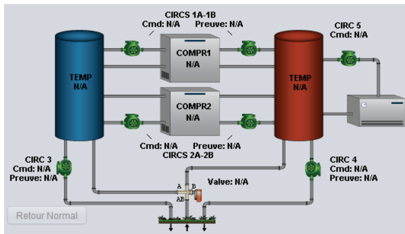
Figure 20 - Séquence à récupération double (double compresseurs démontrés)
