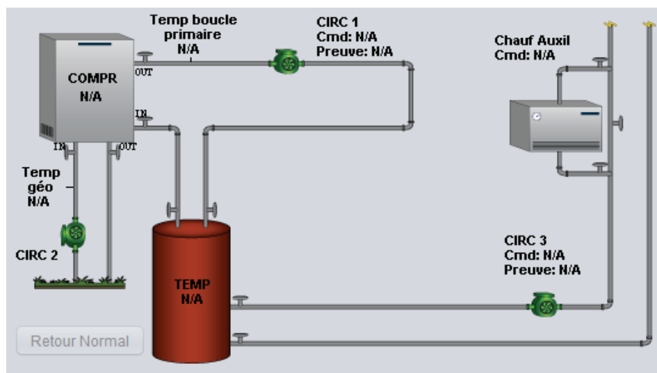
Figure 11 - Séquence de réservoir d'eau chaude simple avec boucle de chaudière ouverte
