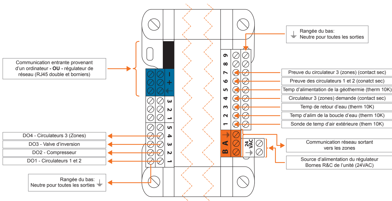
Figure 18 - Identification des entrées et sorties (réservoir d'eau froide simple)
