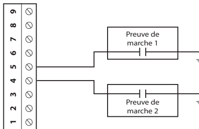
Figure 27 - Raccordement des preuves de marche
