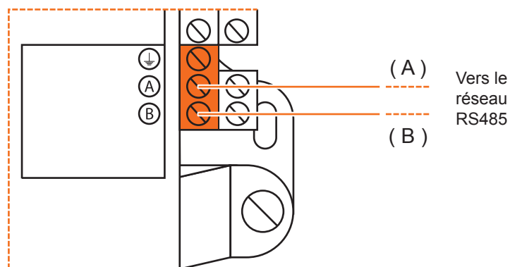
Figure 32 - Raccordement au réseau
