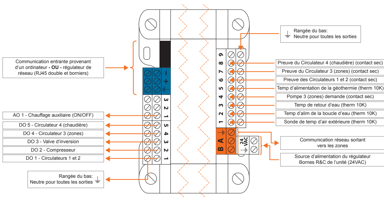
Figure 15 - Identification des entrées et sorties (boucle de chaudière fermée)
