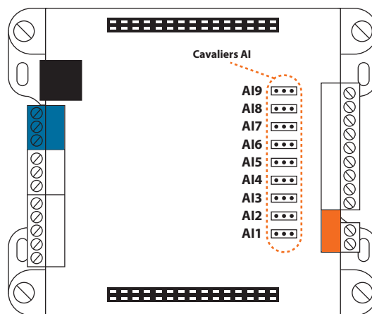
Figure 4 - Localisation des cavaliers internes
