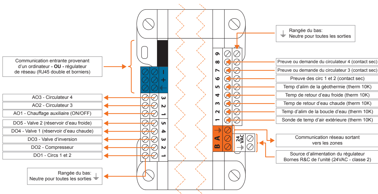
Figure 9 - Identifications des entrées et sorties (réservoir d'eau chaude et froide)
