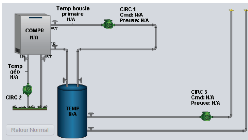
Figure 17 - Séquence simple à réservoir d'eau froide
