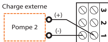
Figure 29 - Raccordement de la sortie analogique 1
