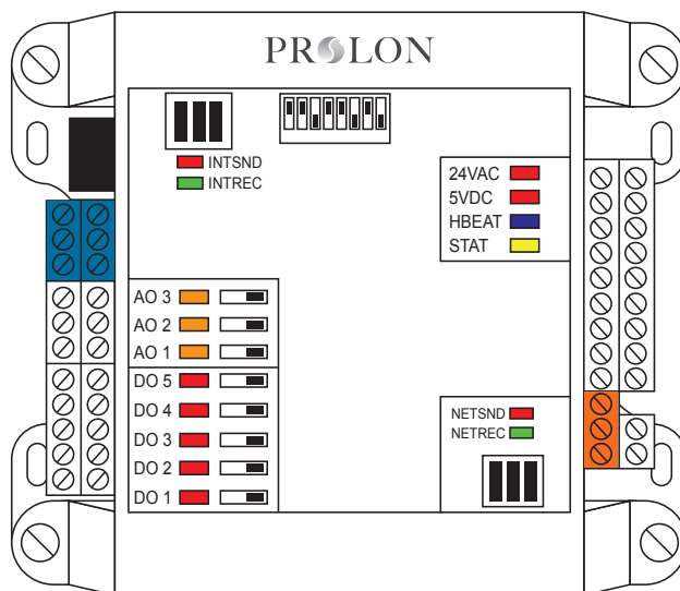
Figure 2 - Identification des témoins lumineux
