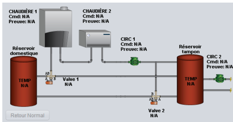
Figure 23 - Séquence de chaudières biénergie
