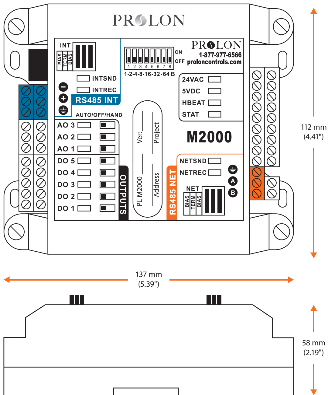
Figure 33 - Dimension du M2000
