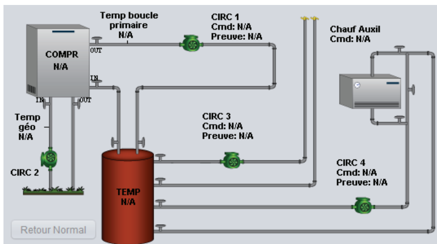
Figure 14 - Séquence simple à réservoir d'eau chaude avec boucle de chaudière fermée
