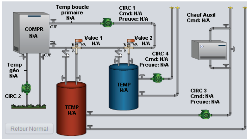
Figure 8 - Séquence de réservoir d'eau chaude et froide
