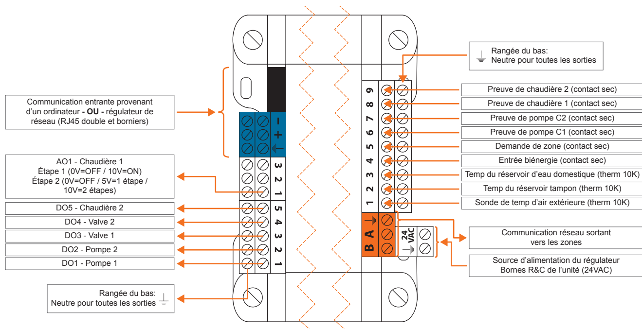
Figure 24 - Identification des entrées et sorties (chaudières biénergie)
