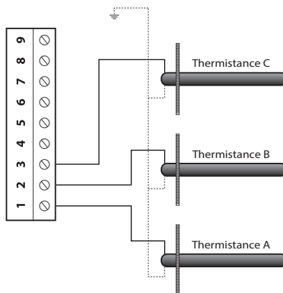
Figure 26 - Raccordement des sondes de température
