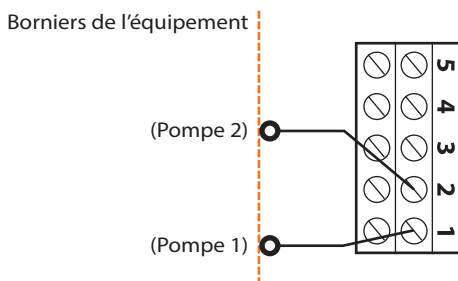
Figure 28 - Raccordement des sorties digitales 1 et 2
