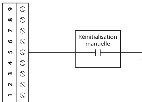
Figure 13 - Raccordement du contact de réinitialisation manuelle
