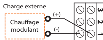
Figure 15 - Exemple de raccordement de la sortie analogique 1
