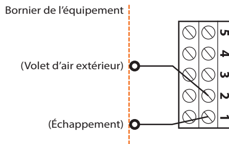
Figure 14 - Exemple de raccordement des sorties digitales 1 et 2
