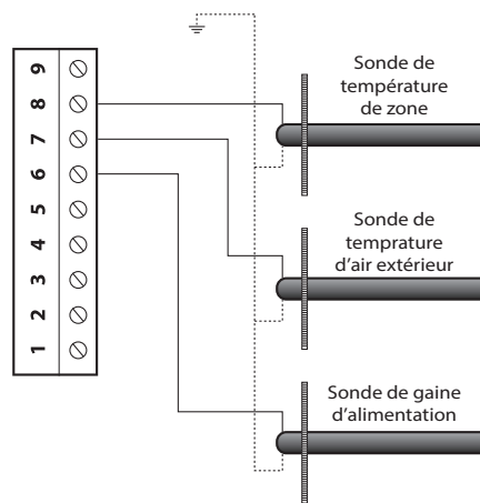
Figure 10 - Raccordement des sondes de température
