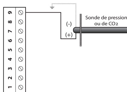
Figure 11 - Raccordement des sondes de pression et de CO 2
