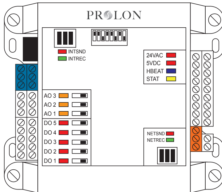
Figure 2 - Identification des témoins lumineux
