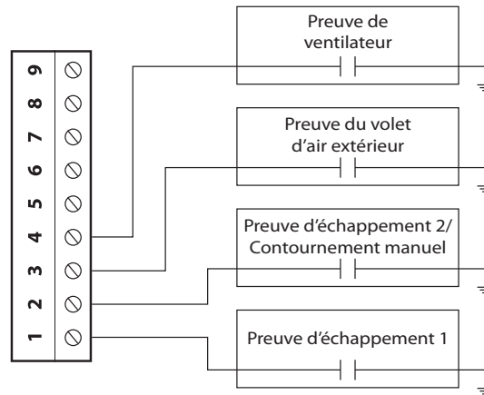
Figure 12 - Raccordement des preuves de marche au régulateur
